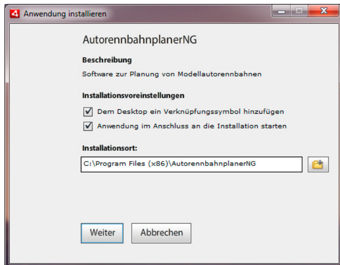
Abbildung 1: Installationsassistent
